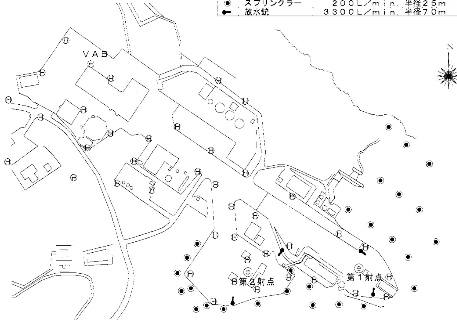
図-2 吉信射点消火設備配置図
