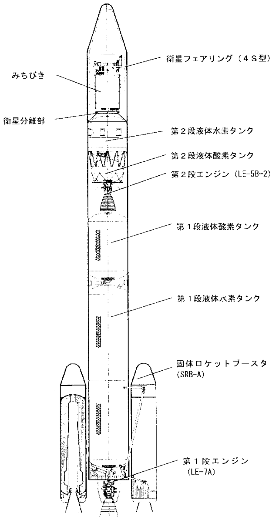
図-1 H-IIAロケット搭載保安物概要 (全段組立)
