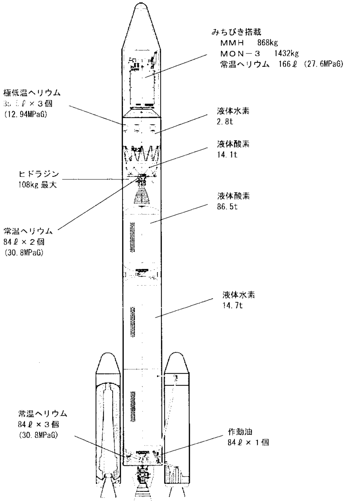
図-1 H-II A ロケット搭載保安物概要 (高圧ガス、危険物等) (2/2)
