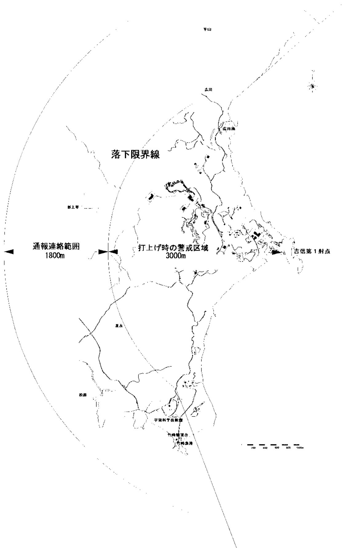
図－4 ガス拡散範囲に係る通報連絡範囲及び落下限界線
