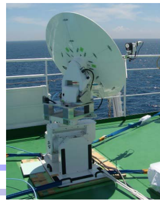
左: 動揺安定台とアンテナ(協力: 東京海洋大)、右: 海洋ロボットMR-X1
