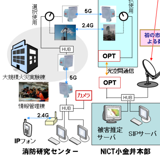
WINDSシンポジウム (H22/2/4,5) デモ・ネットワーク構成図 (防災デモ実験)
