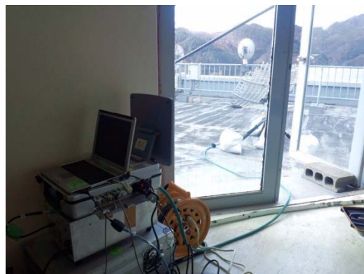
大槌町中央公民館に設置された可搬型通信実験用端末
