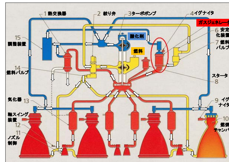
⑤RD-0110エンジン系統図
