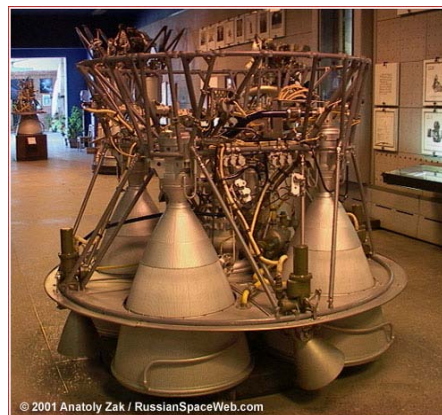
④第3段エンジン(RD-0110)
