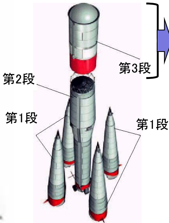
②ソユーズUロケットの構成
