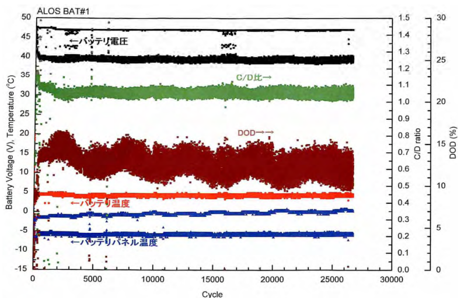
軌道上運用5年間におけるバッテリーの電圧・温度・C/D比・DODの推移
