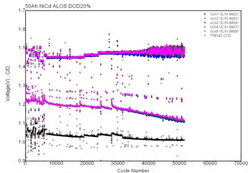
地上運用模擬試験結果(DOD20%@10°C)
