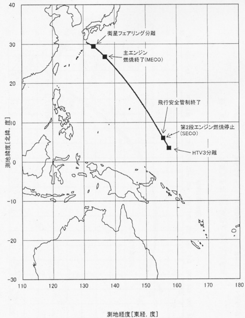
図-6 H-II B ロケット3号機の飛行経路概要 (機体現在位置)
