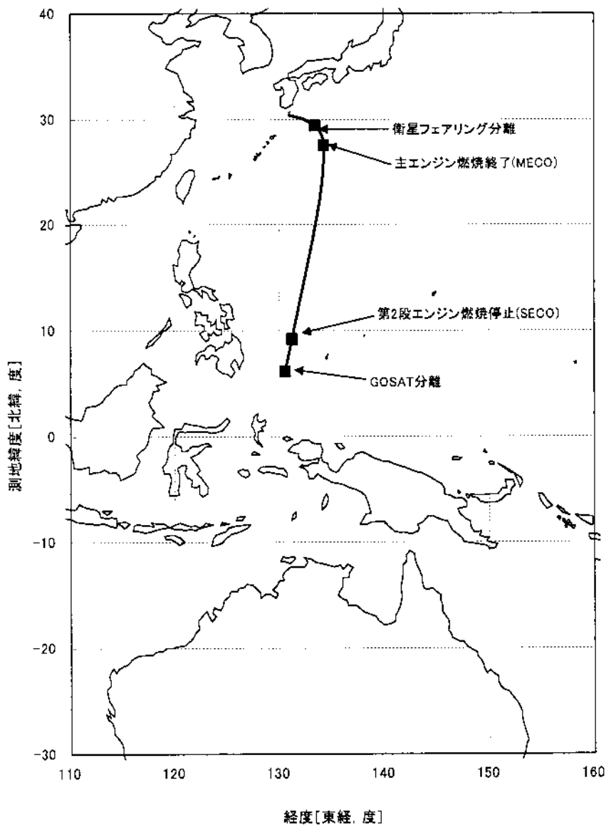
図-6 H-II A ロケット15号機の飛行経路概要(機体現在位置) (1/2)
