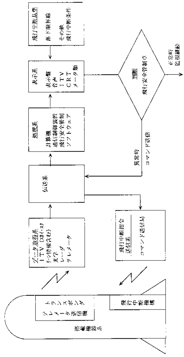
図-9 飛行安全システム概念図
