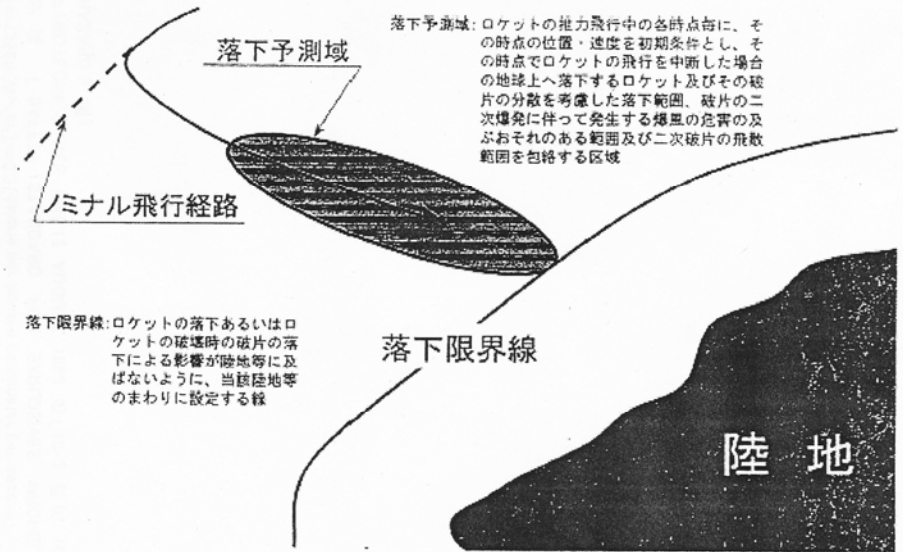
図1 落下予測域と落下限界線
