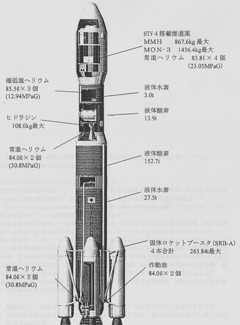
図-1 H-II Bロケット搭載用保安物概要(火薬類、高圧ガス及び危険物)
