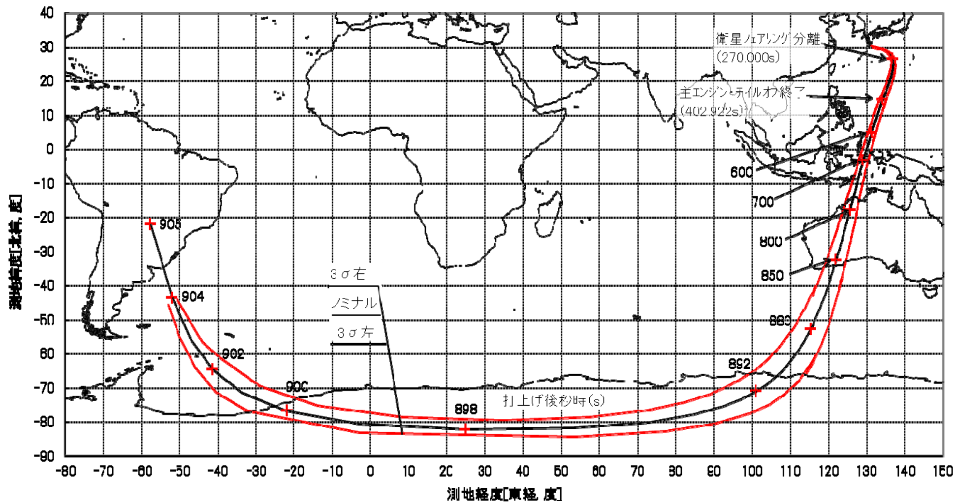
(注) 図5 ロケットの落下予測点軌跡と3σ分散範囲
